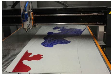
De geprinte en gesealde platen in de juiste vorm frezen
